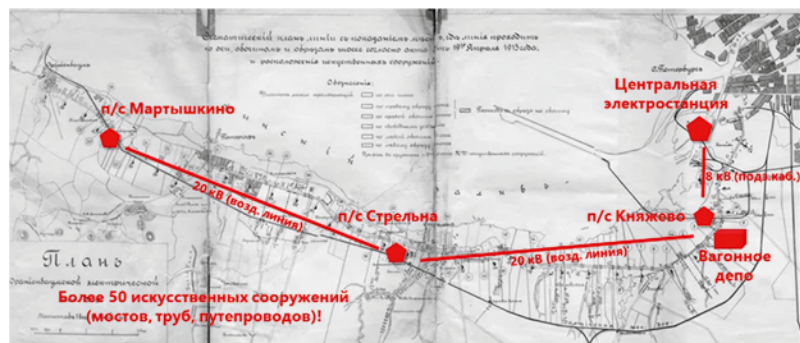
Инфраструктура Ораниенбаумской электрической железной дороги
