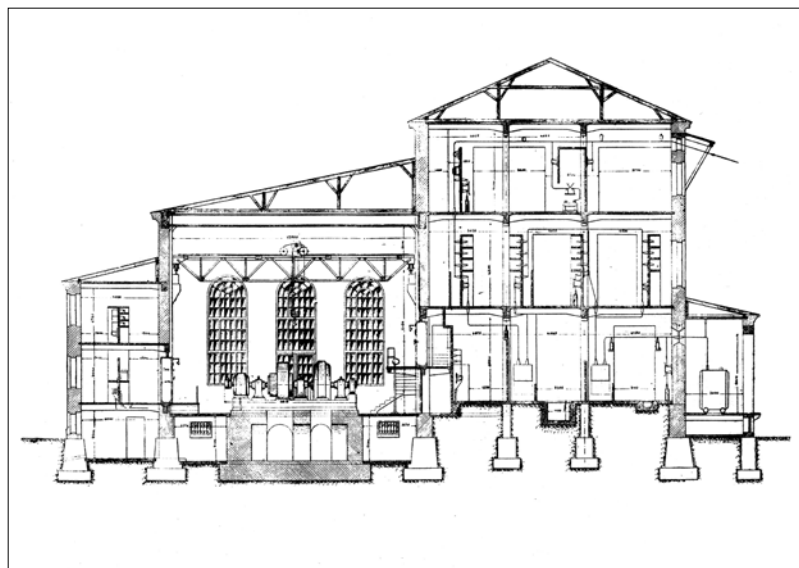
Проект подстанции Княжево (продольный разрез)
